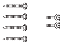
Фиксаторы задней панели (f) (M3.5 × 25) мм, 4EA (g) (M4 × 13) мм, 2EA
