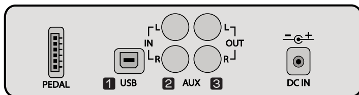
Панель для подключения внешних устройств (на нижней стороне пианино)
